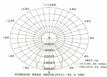
Fotometría para CHB200 con reflector acrílico 70°
