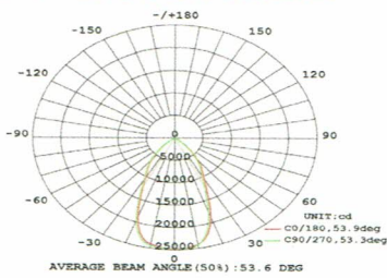
Fotometría para CHB200 con reflector de aluminio 60°
