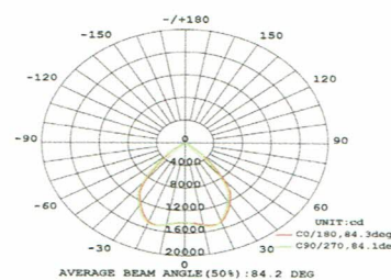
Fotometría para CHB200 con reflector de aluminio de 90°
