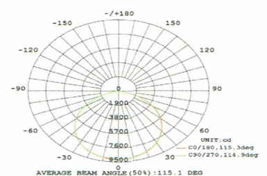
Fotometría para CHB200 sin reflector a 120°
